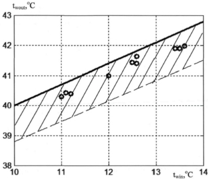
Рисунок 4.8 – Сопоставление расчетных и экспериментальных температурных данных по работе в режиме на входе в аппарат и на выходе: нагрузка – кольца Рашига 25x25x3 мм, H_k = 0,83 м (заштрихована зона 3 %-ного отклонения)
